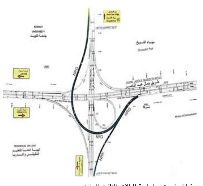
مخطط مشروع ربط طريق المطلاع والدائري السابع
