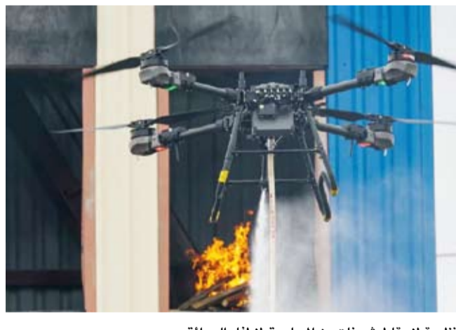
منظومة لإسقاط شحنات من المساحيق لإطفاء الحرائق
